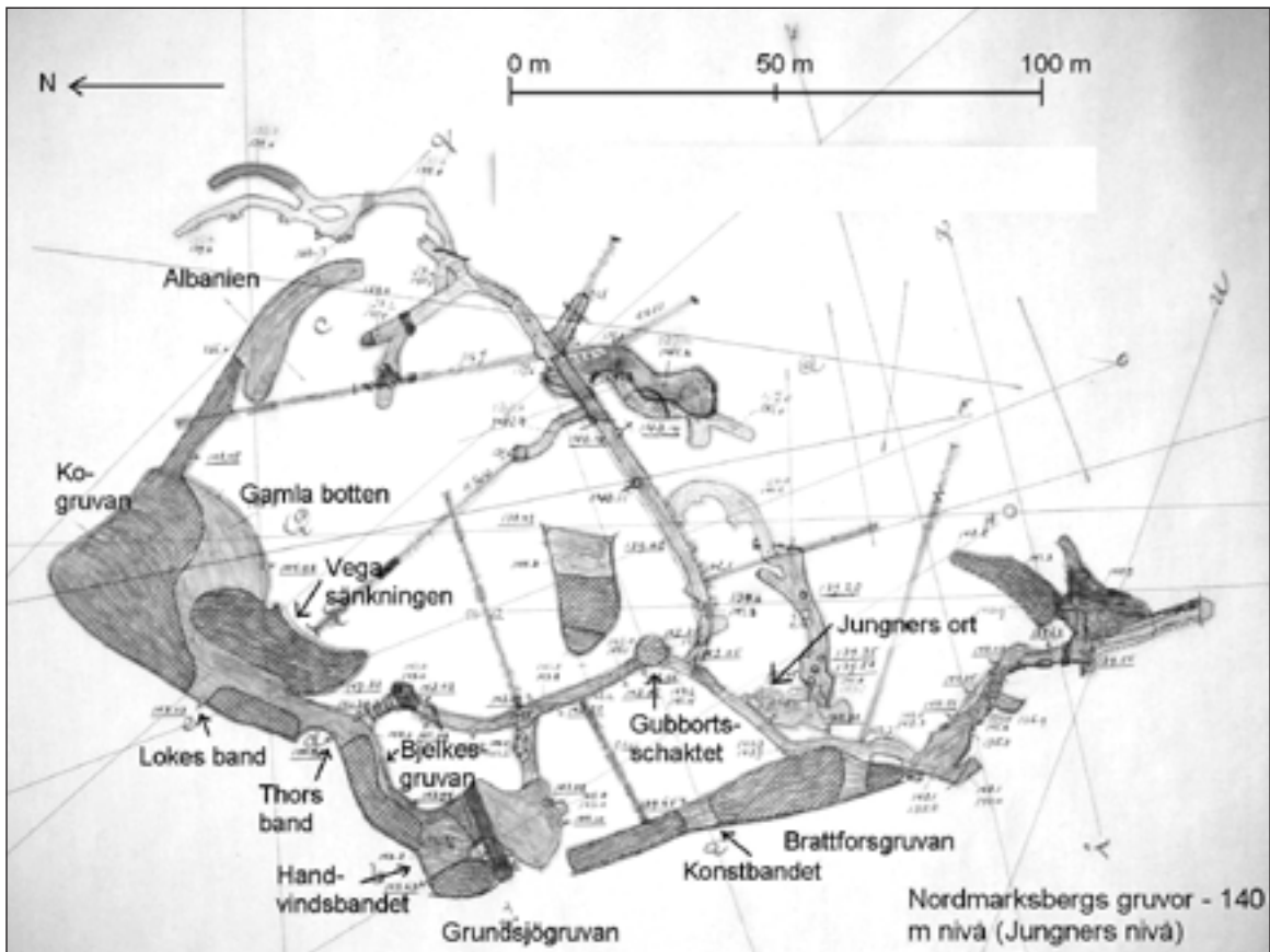
Skiss över Nordmarksbergs gruvor på 140 meters nivå.
