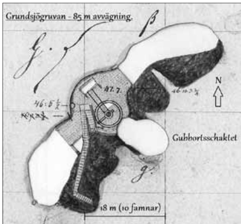
Grundsjögruvan på 85 meters avvägning (djup). Hästvinden som är inritad på kartan här var den som låg djupast i gruvan. Här syns också trärampen som hästarna gick upp och ned på. Notera också det stora trägolvet som byggts över det öppna rummet vilket hästen gick runt på dagarna i ända. Det blev nog en hel del hästskit i gruvan att ta reda på under ett år!
